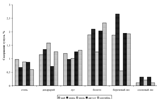
Рис. 1. Изменение содержания гумуса в теплый период года
