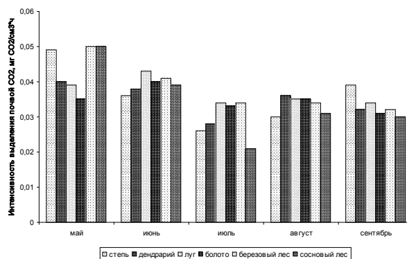
Рис. 6. Изменение интенсивности выделения углекислого газа в почвах Ботанического сада в теплый период года
