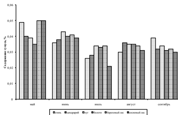
Рис. 2. Изменение содержания гумуса в биотопах Ботанического сада
