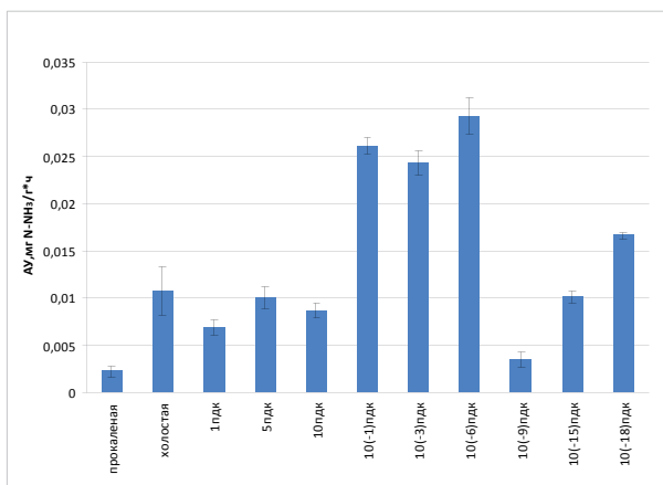
Рис. 2. Активность уреазы почвы
