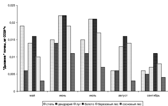
Рис. 4. Изменение «дыхания» почвы в биотопах Ботанического сада
