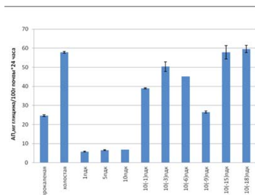
Рис. 1. Активность протеазы почвы, загрязненной МФК
