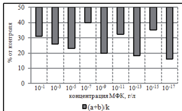
Рис. 4. Изменение отношения суммы хлорофиллов (a+b) к содержанию каротиноидов в листьях проростков кукурузы в зависимости от концентрации МФК
