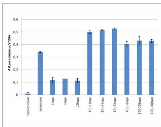
Рис. 3. Активность почвенной инвертазы
