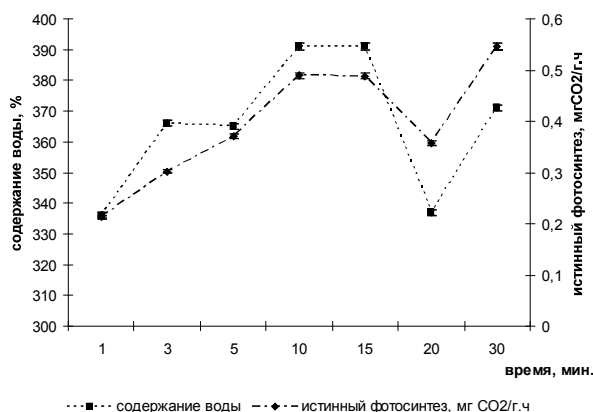
Рисунок 5 – Динамика истинного фотосинтеза в зависимости от поглощения воды побегами Sphagnum palustre
